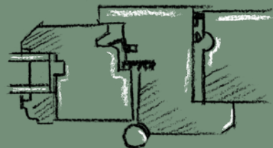
Dormant rénovation pour pose sur bâti existant conservé
