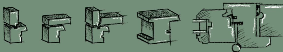
Tapée d'isolation ou volet roulant Tapée persienne Tapée persienne + isolation Rainure à brique Dormant rénovation pour pose sur bâti existant conservé
